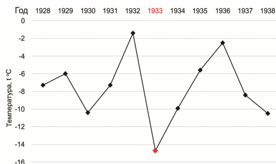
Рисунок 8. Средние значения температуры декабря в 1928-1938 гг. в г. Москве Figure 8. Average values of December temperature in 1928-1938 in Moscow
